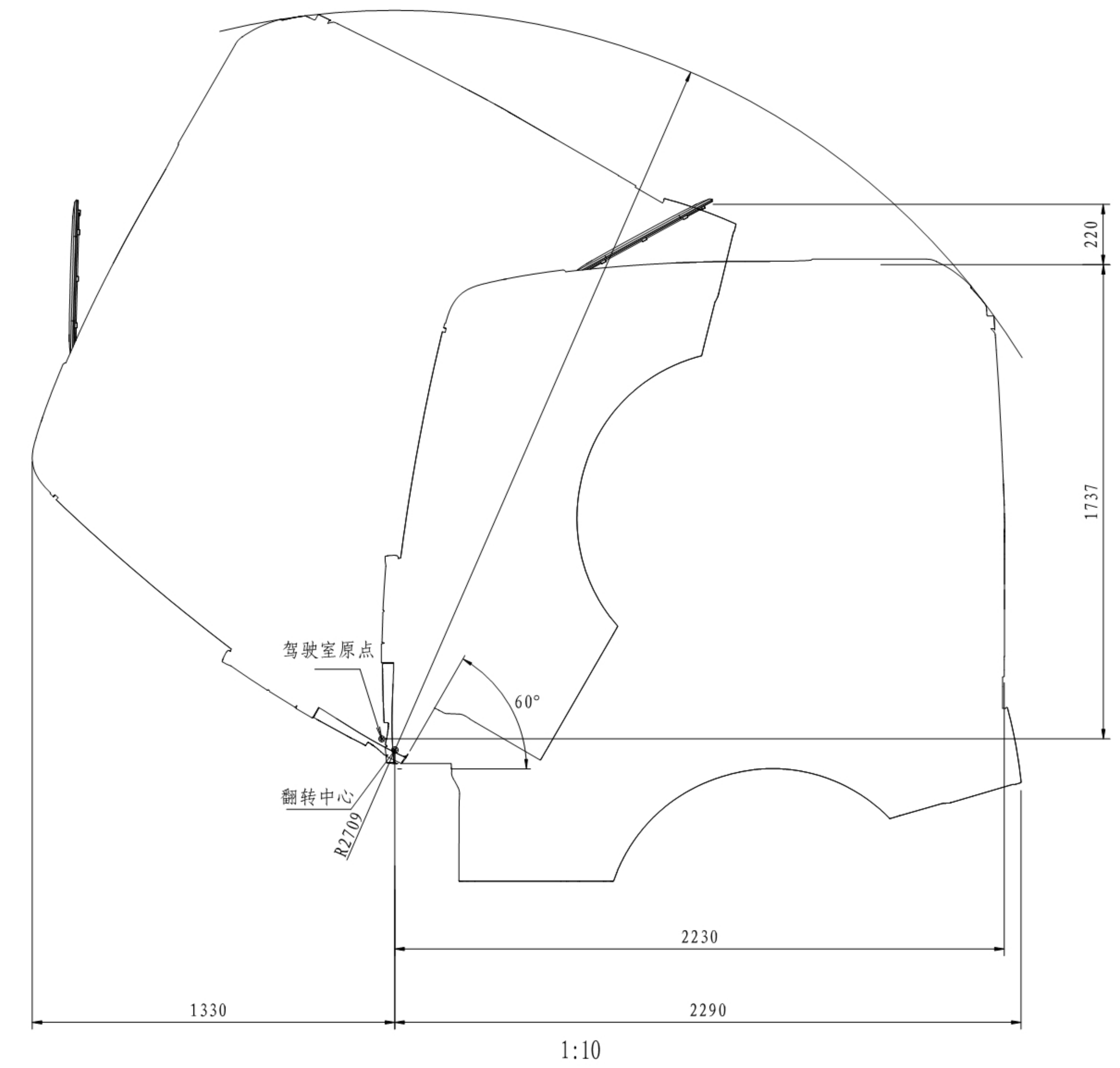
TX-F驾驶室翻转示意图 1:10
